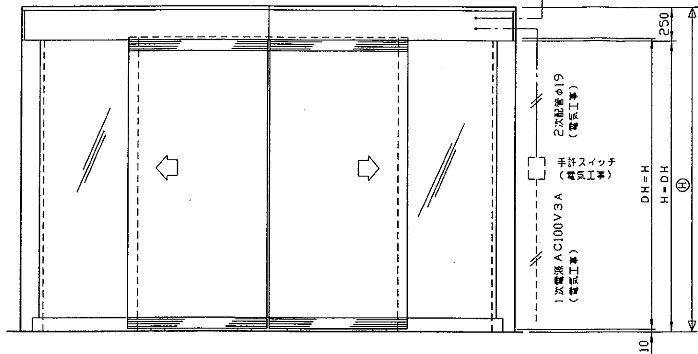
内観姿図
